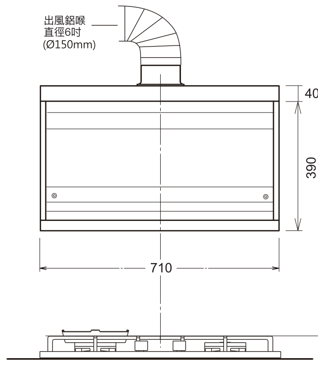
Front view 正面圖
