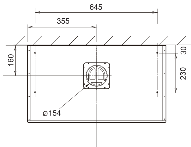
Top view 機頂平面圖
