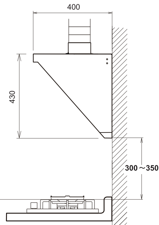
Side view 側面圖
