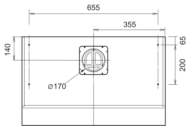
Top view 機頂平面圖
