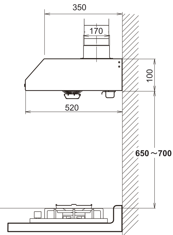
Side view 側面圖
