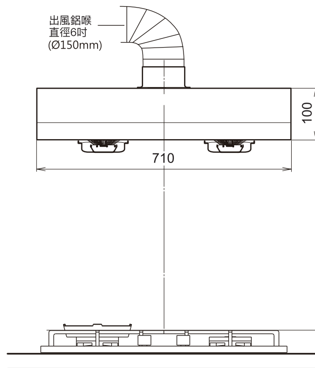
Front view 正面圖
